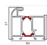
Rysunek techniczny
